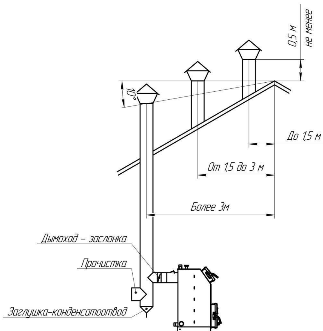
Рис. 2 Варианты установки дымовой трубы
